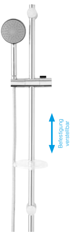
Brausestangenset Handbrause Ø 9,5 cm , Brausestange 90 cm, Brauseschlauch 150 cm, Seifenschale, Chrom
