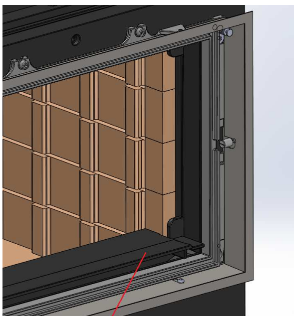
Luftleiste
