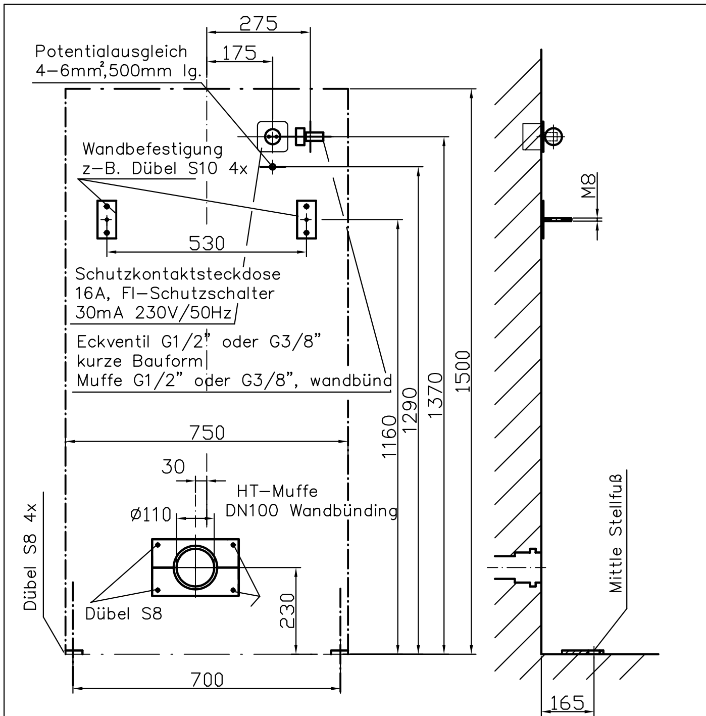
Wandvorbereitung für Montage Lift WC100, Abflussschlauch DN100
